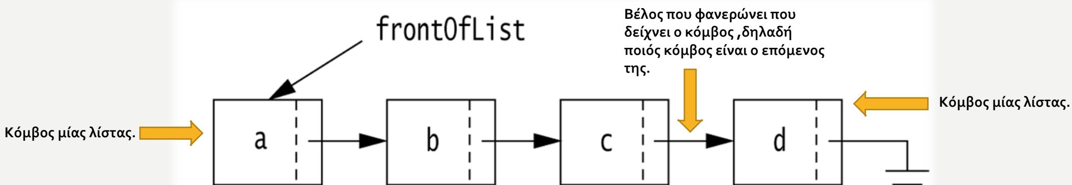
Μία λίστα με τέσσερις κόμβους.
